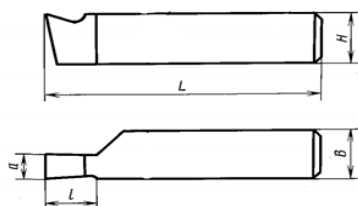
Резец прорезной
